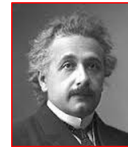
A.Einstein 1916
