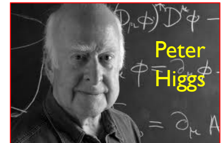
+ il bosone di Higgs
