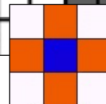
Intorno di von Neumann
